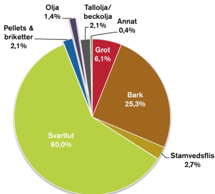
Figur 12. Bränslefördelning för elproduktion i skogsindustrin 2020
